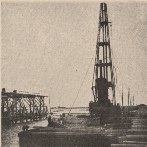
Kafar, parowy zmontowany na pontonie (do wbijania pali)
