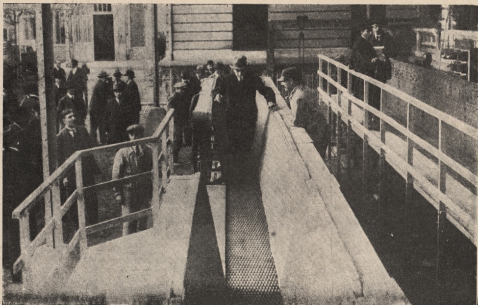
Jeden z chodników ruchomych, które wkrótce znajdą zastosowanie na ulicach Paryża. Aparat Bouchel'a, mogący posuwać chodnik z szybkością 9 kłm. na godzinę
