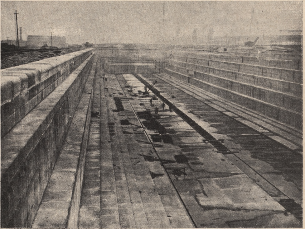
Suchy dok długości 250 metrów, w którym pomieścić można statek 20 tys. tonowy
