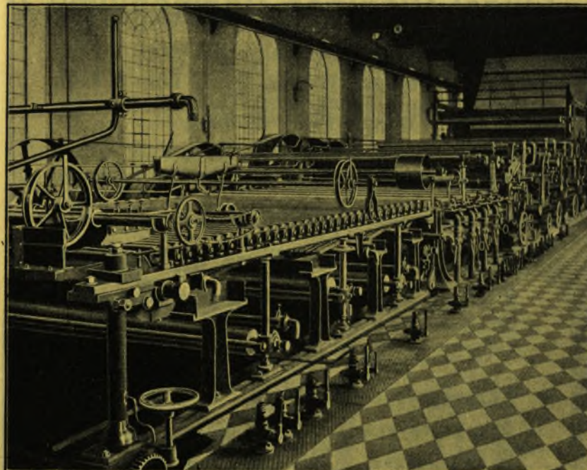
Siebpattie einer von mir ausgeführten Druckpapiermaschine.
