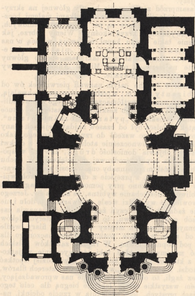
Rys. 52. Rzut poziomy kościoła O.O. Dominikanów.
