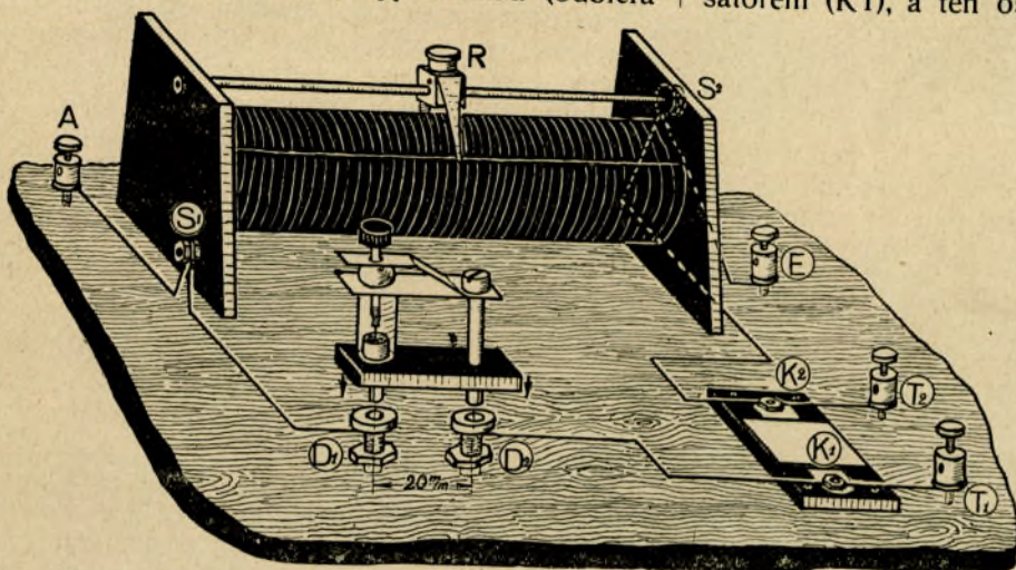
Fig. 1. Najprostszy radiotelefoniczny aparat odbiorczy.
