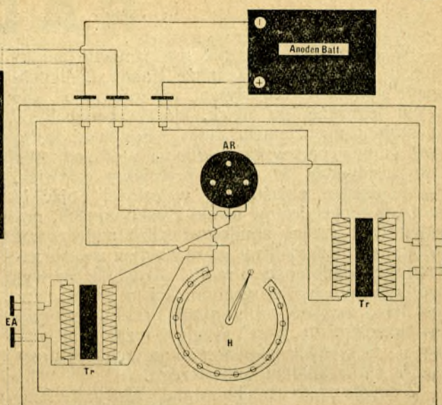
Fig. 4. Wzmacniacz detektora.
