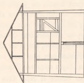
Querschnitt
