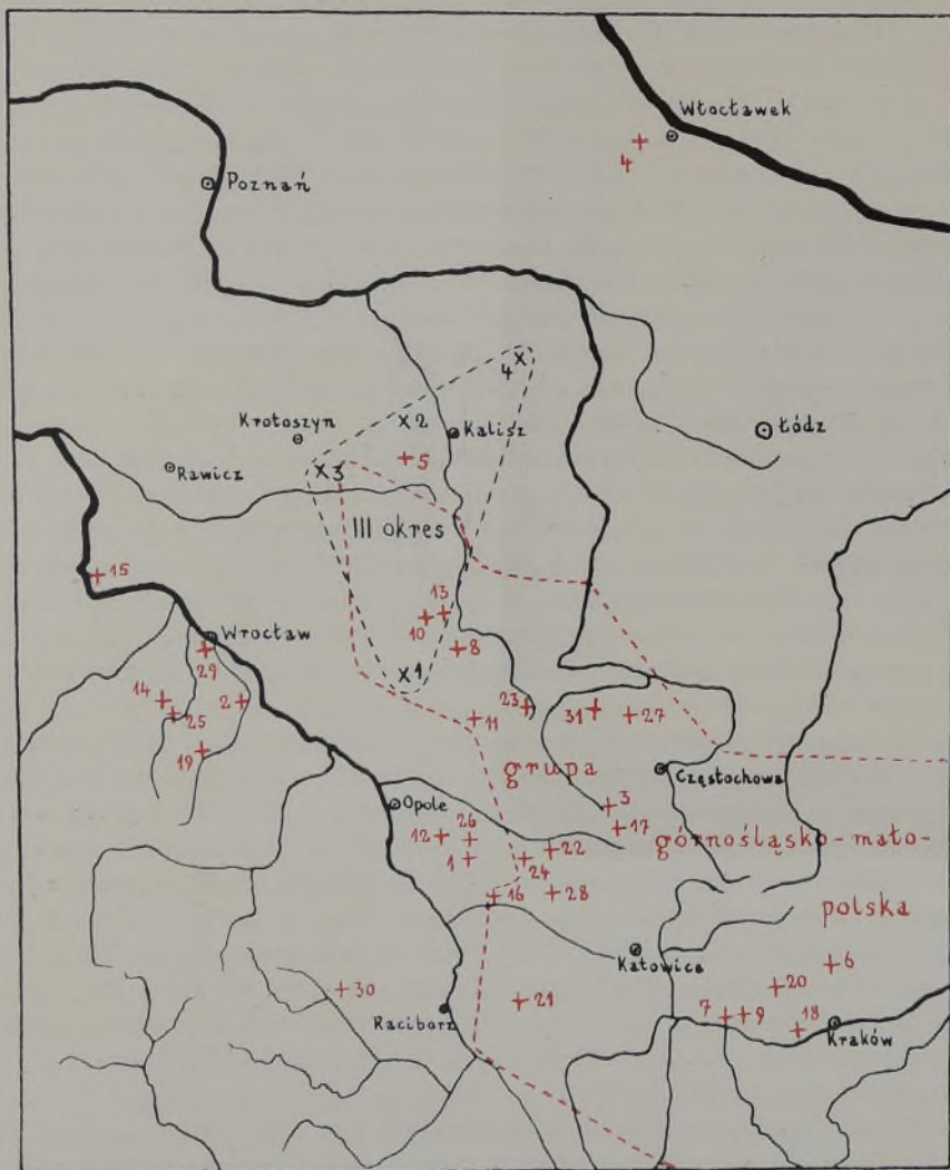
Ryc. 1. Mapa grobów szkieletowych kultury łużyckiej na Śląsku i w Polsce zachodniej w III i V okresie epoki brązowej i okresie Hallstatt C. Skala 1:2,500,000.
