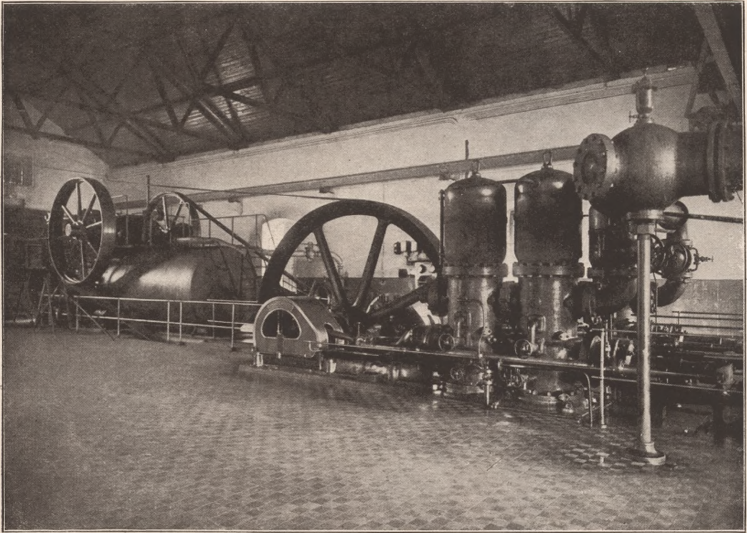
Neue Pumpenanlage Merzdorf
