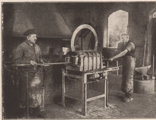
Gasschmiedeofen „Universal“, — D. R. P. a.
