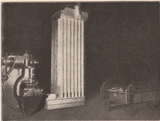
Gasbeheizter Luftheizer für 400 000 WE i. d. St., im Bau begriffen. — D. R. P. a. —
