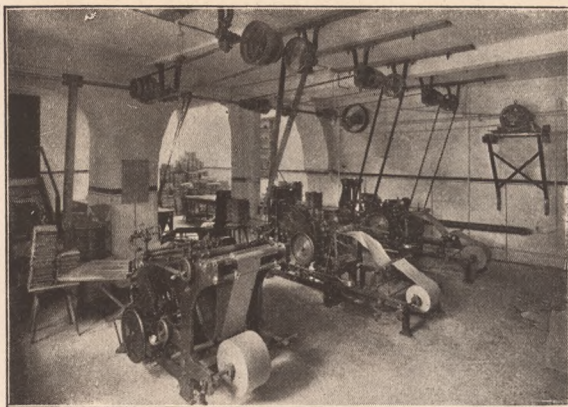
Teilansicht des Maschinensaales
