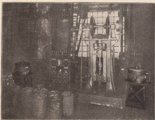
Schmiedepresse für Massenfabrikation mit zwei kontinuierlich arbeitenden Gasglühöfen D. R. P. a.
