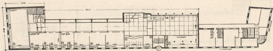
Plan I piętra.
