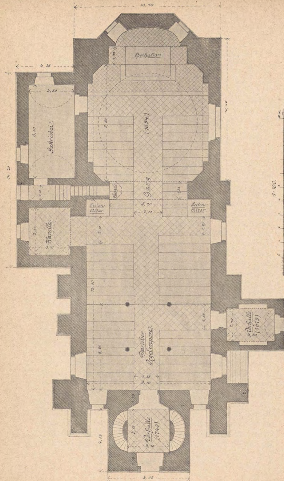
Grundriß der St. Georg-Kirche zu Rückerwalde.
