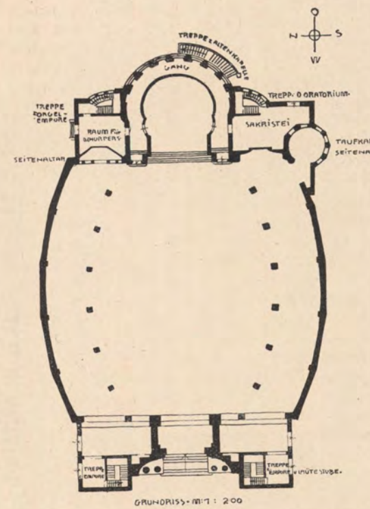
MOTTO »ORCHIDEEN« GRUNDRIß Nr. 27, Text S. X, vgl. Nr. 24 und 28
