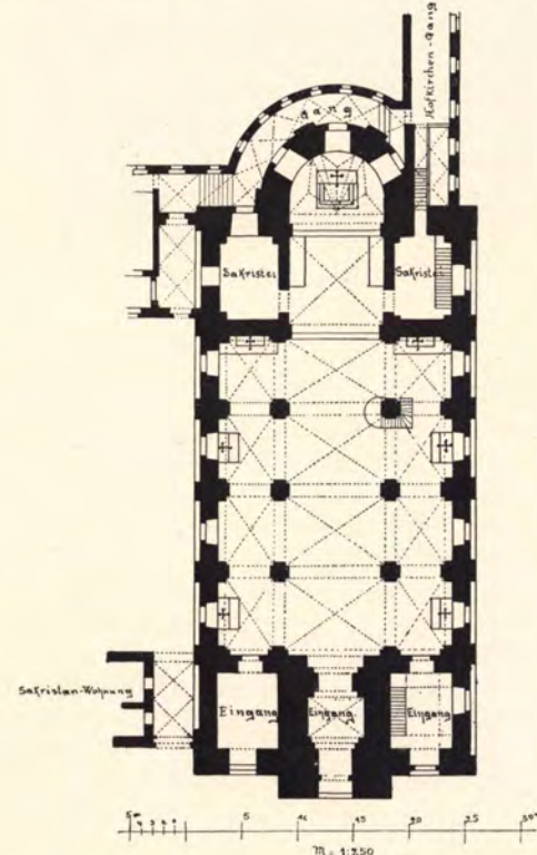
GRUNDRISS DER HOFKIRCHE IN NEUBURG a. D.
