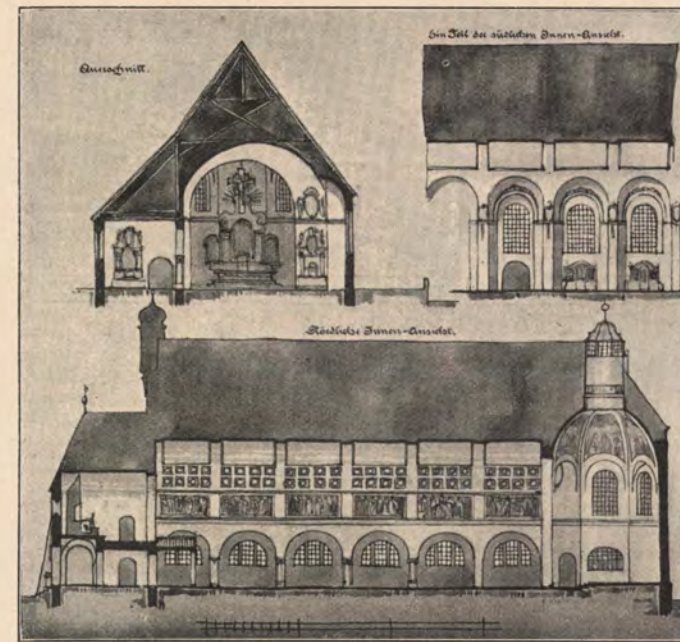
MOTTO »ZWEISCHIFFIG« Nr. 15, Text S. VII-X, vgl. Nr. 12-14
