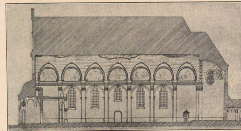
MOTTO »SKABIOSE« LÄNGENSCHNITT Nr. 21, Text S. X, vgl. Nr. 25, 26, 29
