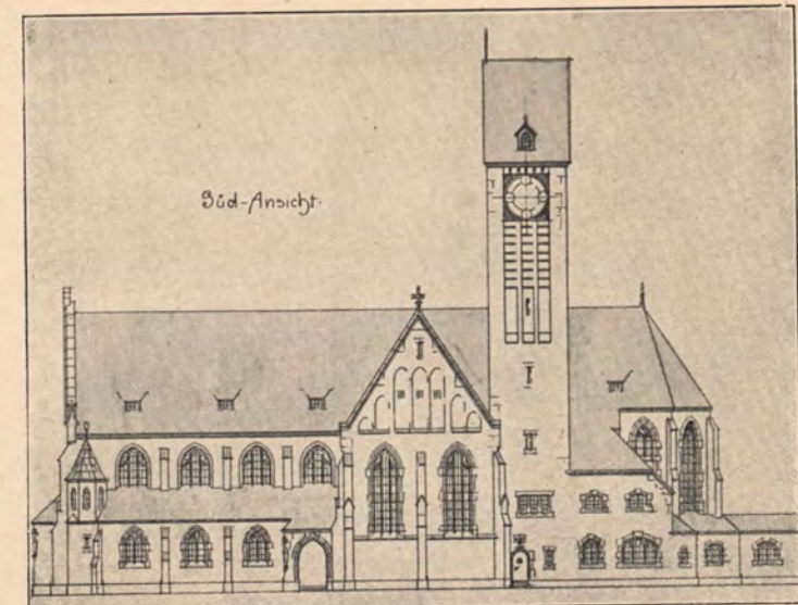
MOTTO »QUERSCHIFF« SÜDLICHE AUSSENANSICHT Nr. 19, Text S. XII, vgl. Nr. 18 und 20
