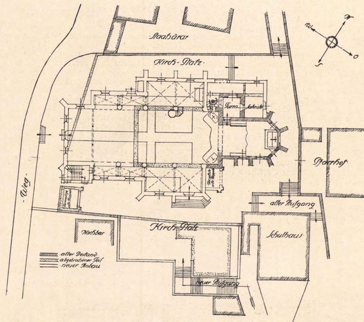
ERWEITERUNG DER WALLFAHRTSKIRCHE ZU HÖCHBERG IN UFR. DURCH ARCHITEKT RUDOLF HOFMANN IN WÜRZBURG. ANBAU WEISS. VGL. ABB. S. 219
