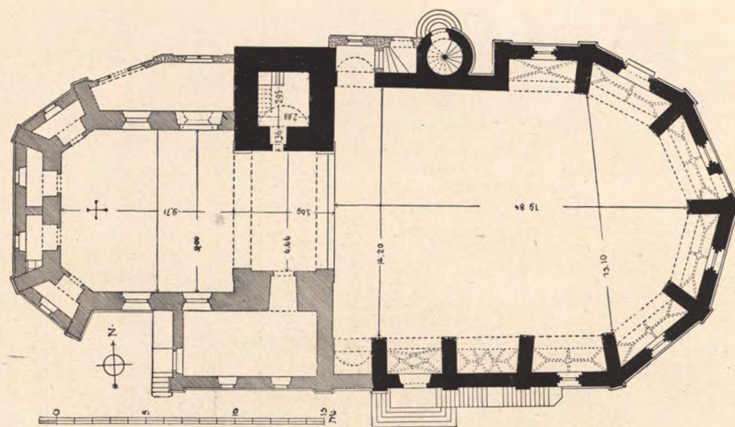
STADTPFARRKIRCHE ZU DETTELBACH IN UNTERFRANKEN. ERWEITERUNG DURCH UMKEHRUNG DES CHORES NACH WESTEN. ANBAU SCHRAFFIERT. VGL. ABB. S. 213 UND 215. — Text S. 208
