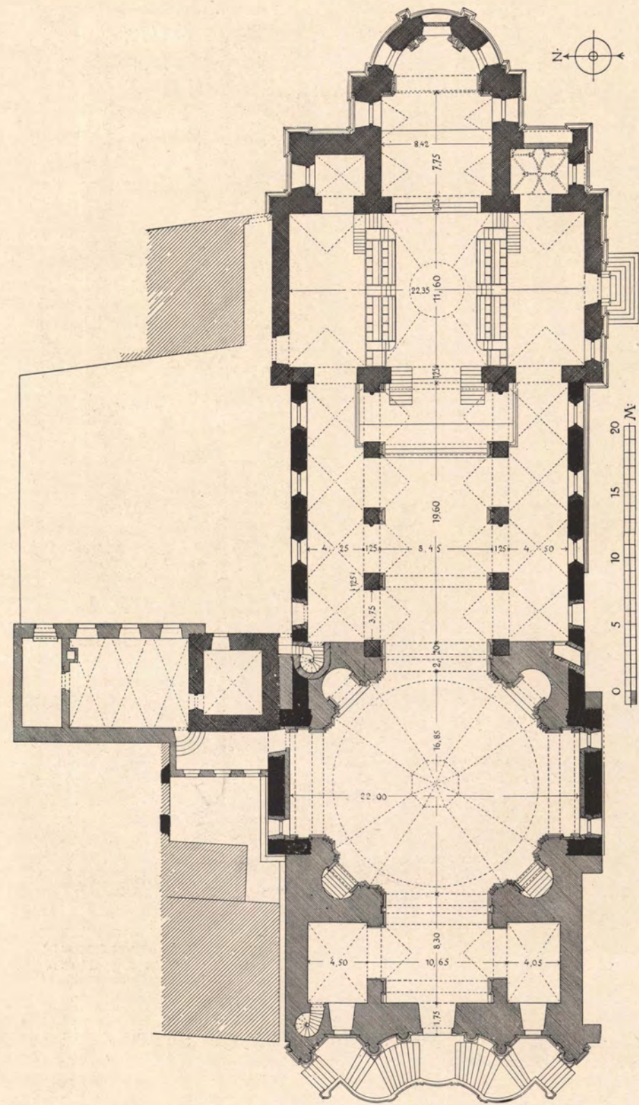
NEUMÜNSTER ZU WÜRZBURG. ERWEITERUNG DURCH ZENTRALBAU IN DER AXSENVERLÄNGERUNG. DIE ÄLTESTEN TEILE SCHWARZ, DIE UMBAUTEN KREUZWEISE, DIE ERWEITERUNGSBAUTEN EINFACH SCHRÄFFIERT. — Text S. 205
