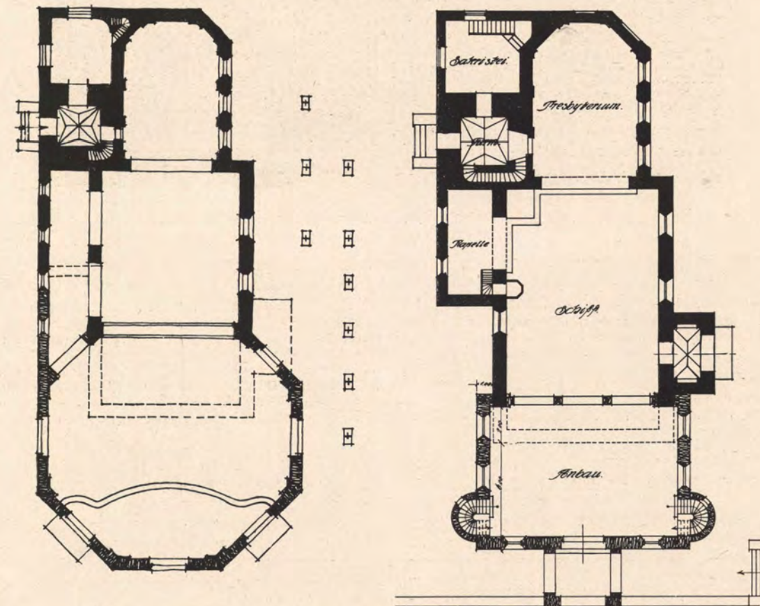
RICHARD BERNDL, ERWEITERUNG DER KIRCHE IN GÜNZELHOFEN. — ERSTES PROJEKT SIEHE GRUNDRISSE LINKS, AUSGEFÜHRTES PROJEKT SIEHE GRUNDRISSE RECHTS
